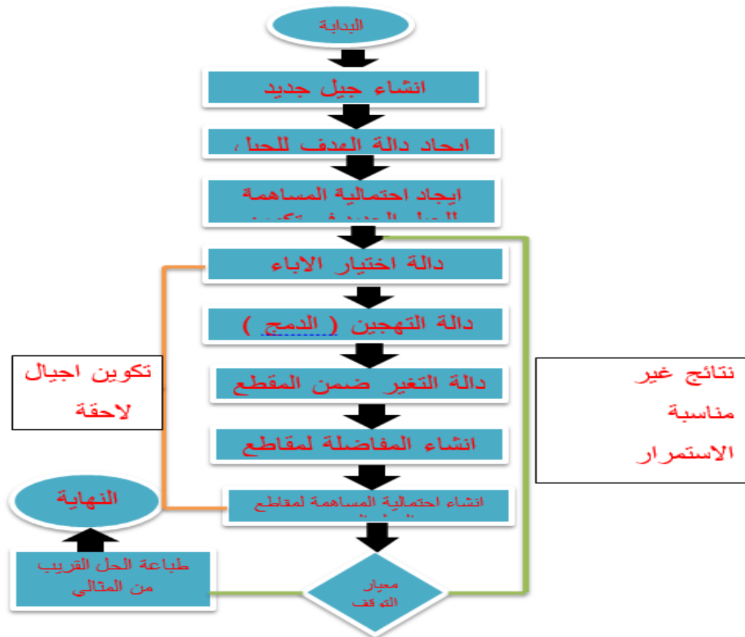
الشكل (2) المخطط العام للخوارزمية الجينية من
