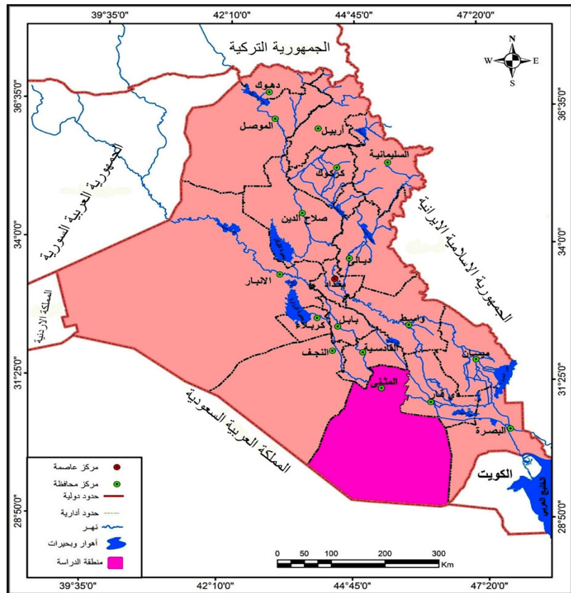
الخريطة (١) موقع منطقة الدراسة من العراق
